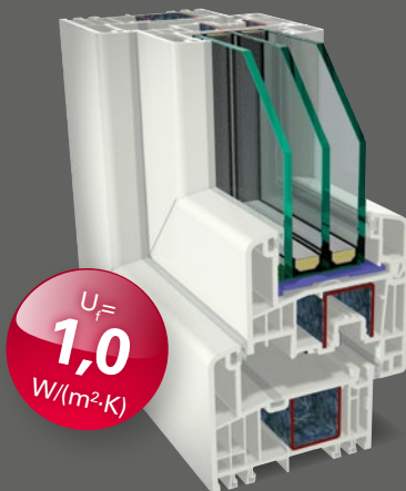
Schmäler Rahmen mit Flügel
