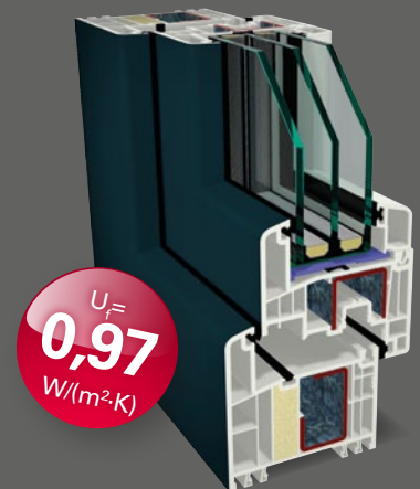
Bester Wärmedämmwert mit hohem Blendrahmen durch Einsatz von IKD®.
