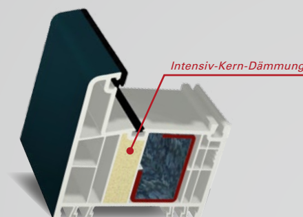
Blendrahmen mit ausge-schäumter IKD®-Kammer.
