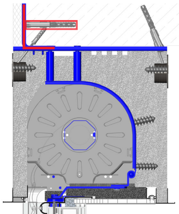
Statikkonsole und Befestigungsset (optional) für Revision innen (Rot dargestellt: optionales Zubehör)
