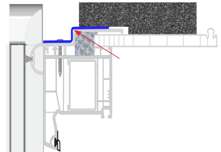
Z- Stahlverstärkungsseisen.
