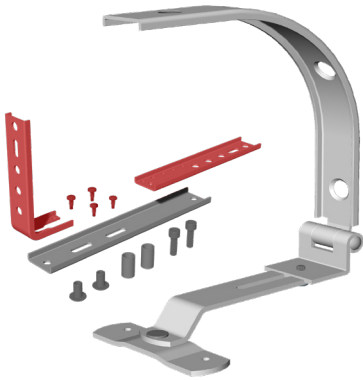
Statikkonsole und Befestigungsset (optional) für Revision innen (Rot dargestellt: optionales Zubehör)
