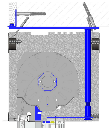
Statikkonsole und Befestigungsset (optional) für Revision außen und Raffstore
